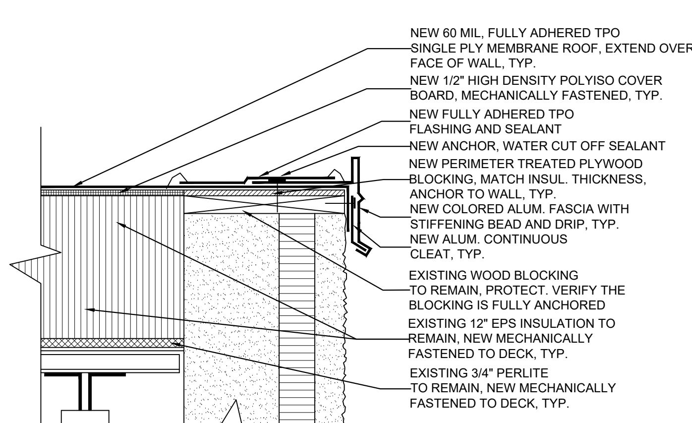
1 18 EXISTING ROOF EDGE DETAIL Scale: 1-1/2" = 1'-0"
